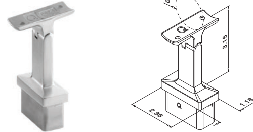
MOD 4719 - □ 2.36" x 1.18" x 0.1"
