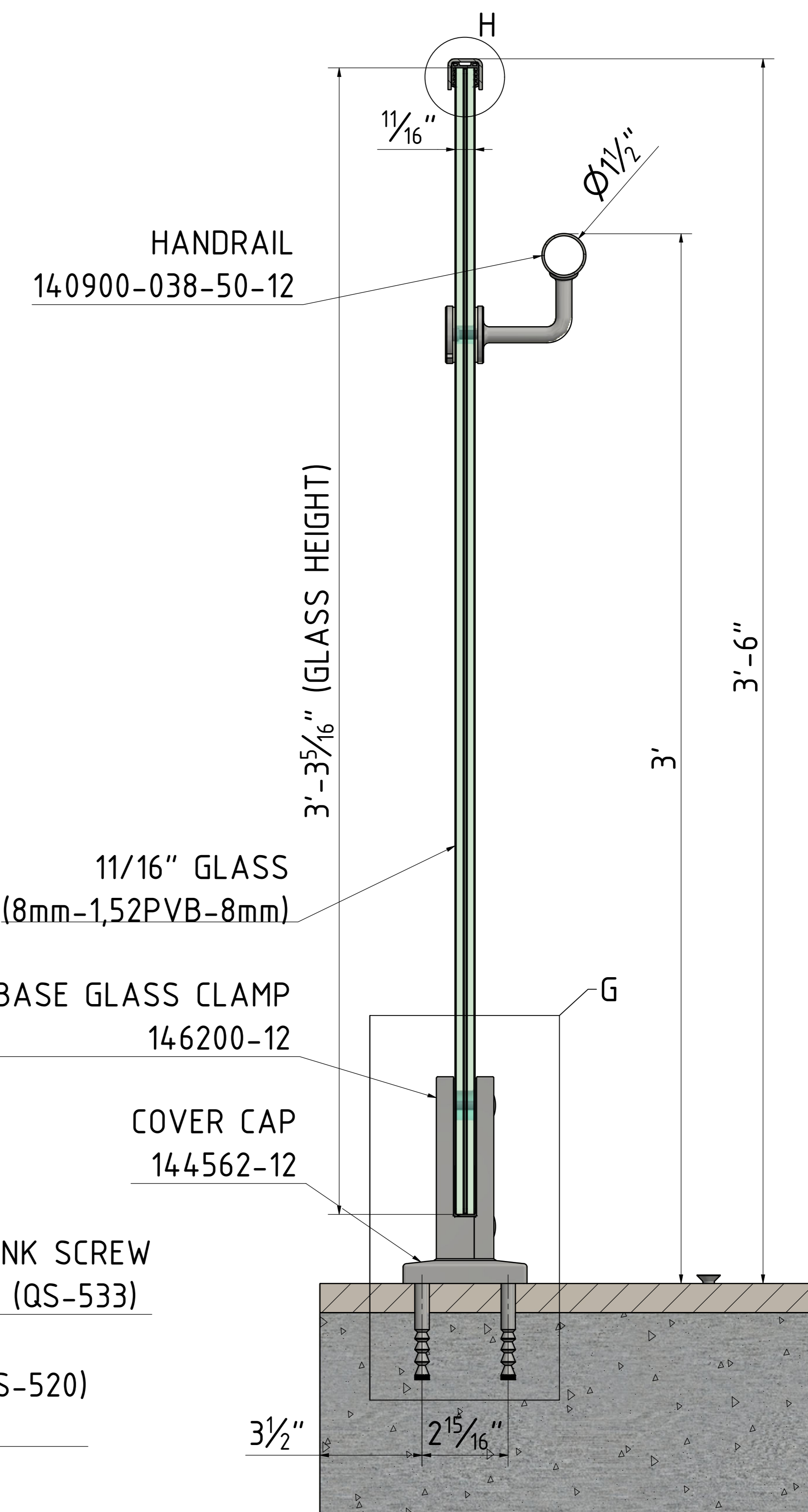
D-D ( 1 : 3 )
