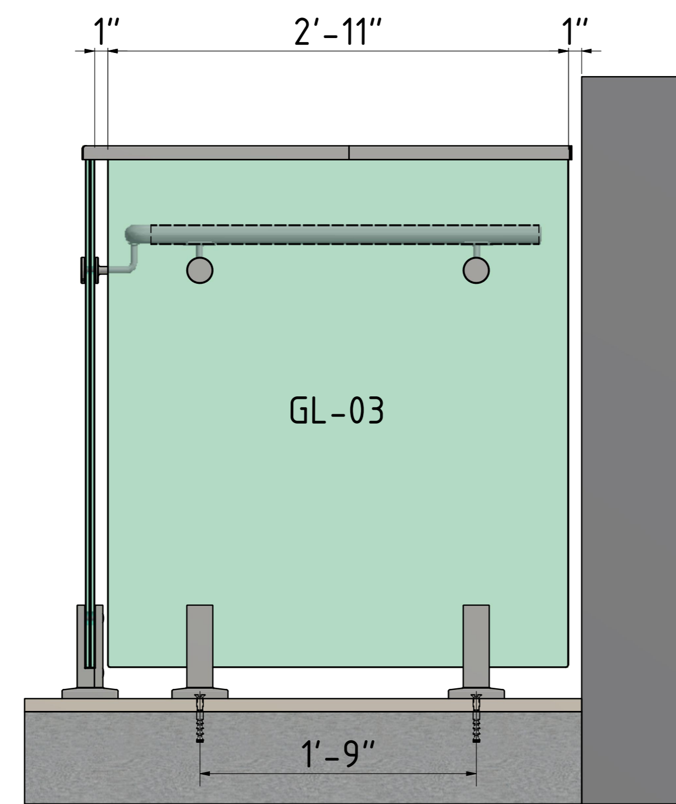
C ( 1 : 7,5 )
