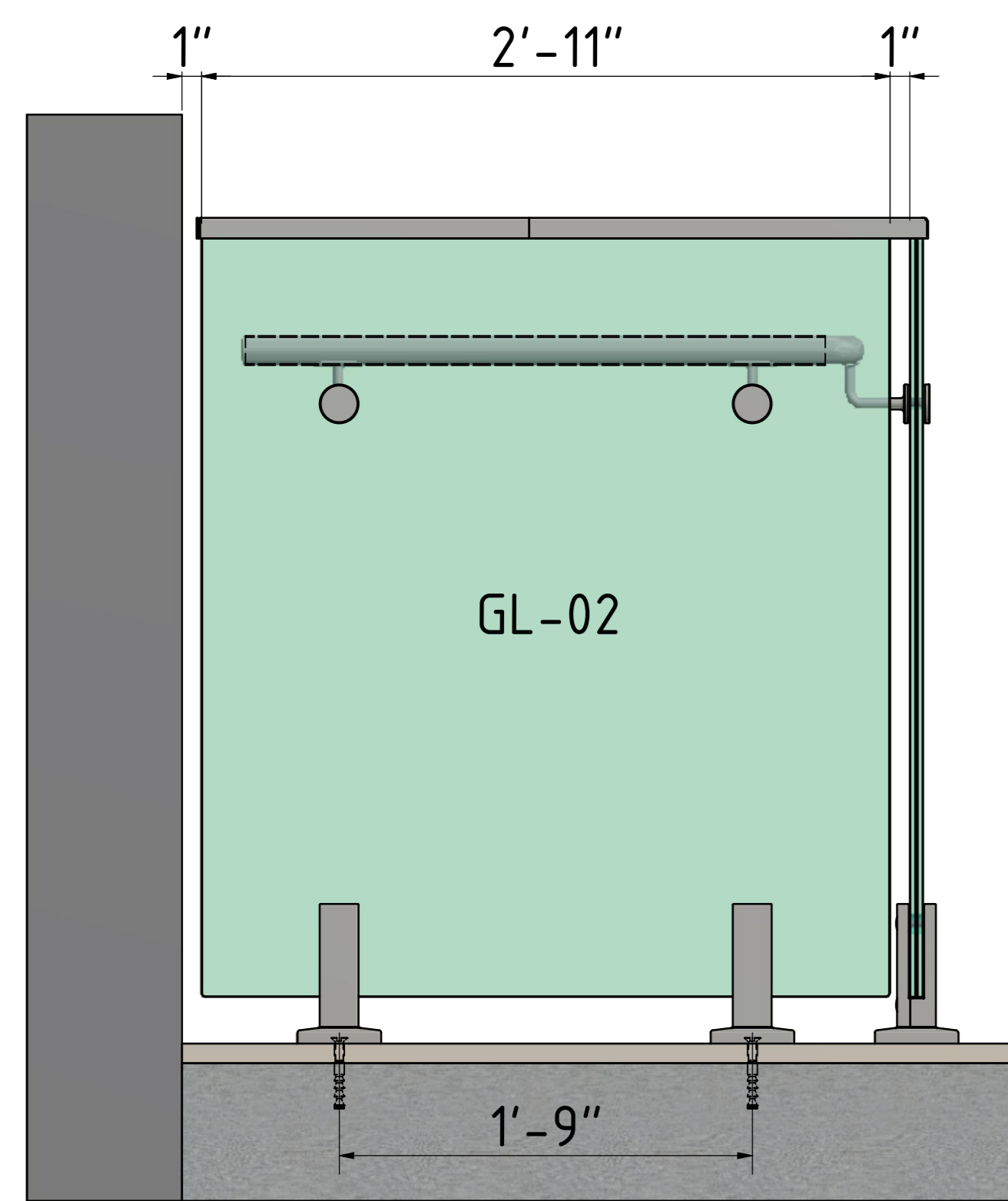
B ( 1 : 7,5 )
